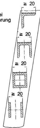
Beispiel von rutschhemmenden Sprossenquerschnitten mit einer Auftrittstiefe von mindestens 20 mm
